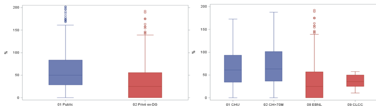
Dispersion statistique
